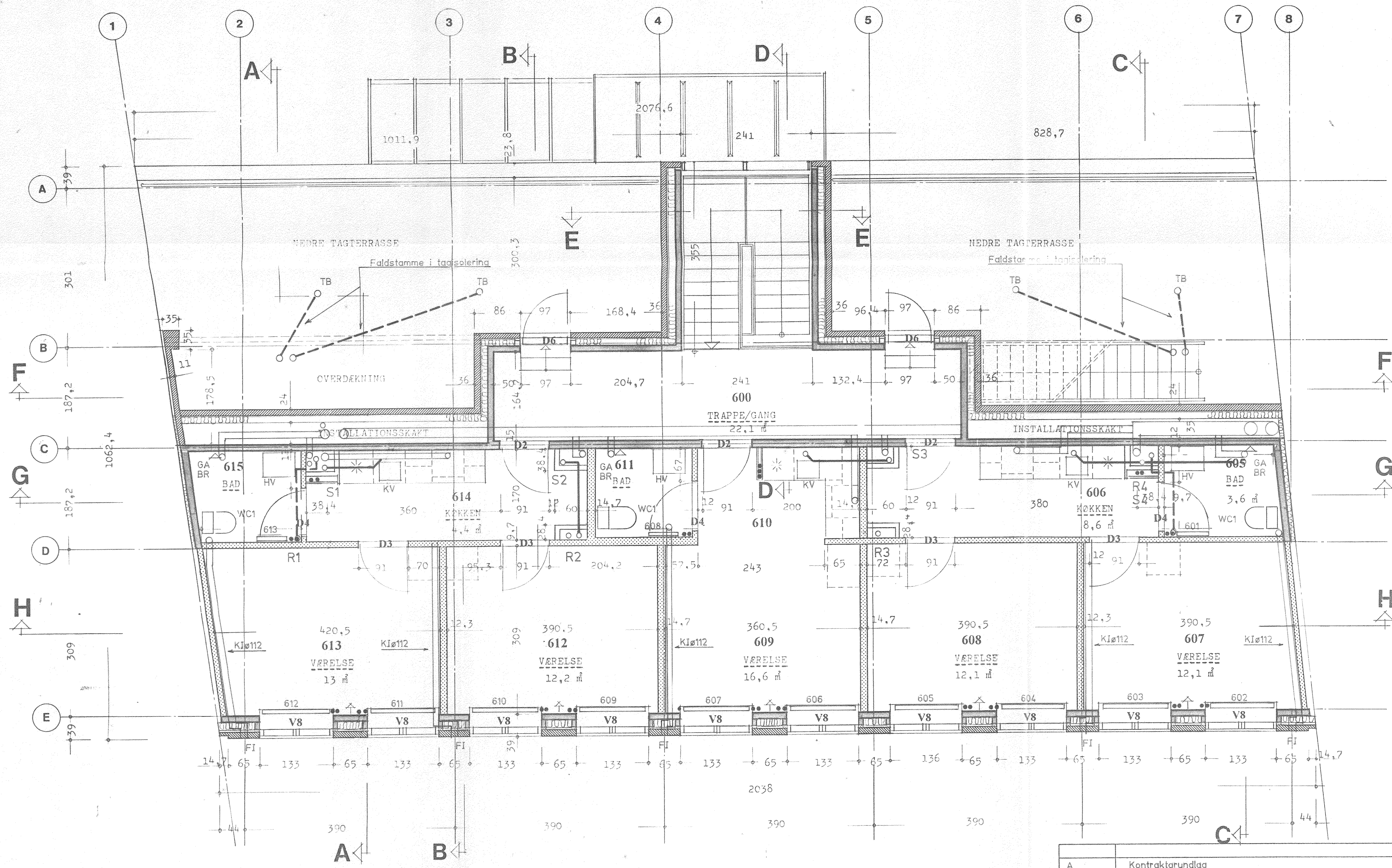
PLAN AF 4. SAL
