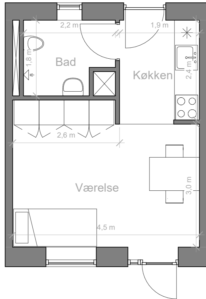
Type 10 - Stueetage
