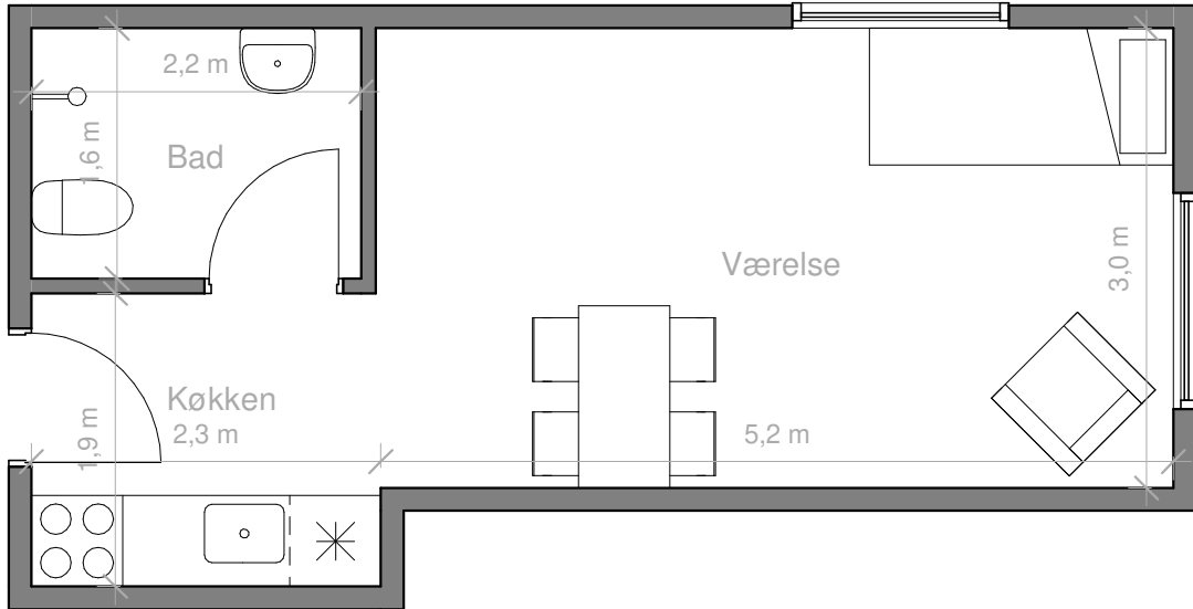
Type 11 Stuen, lejl. 18 1. sal, lejl. 18
