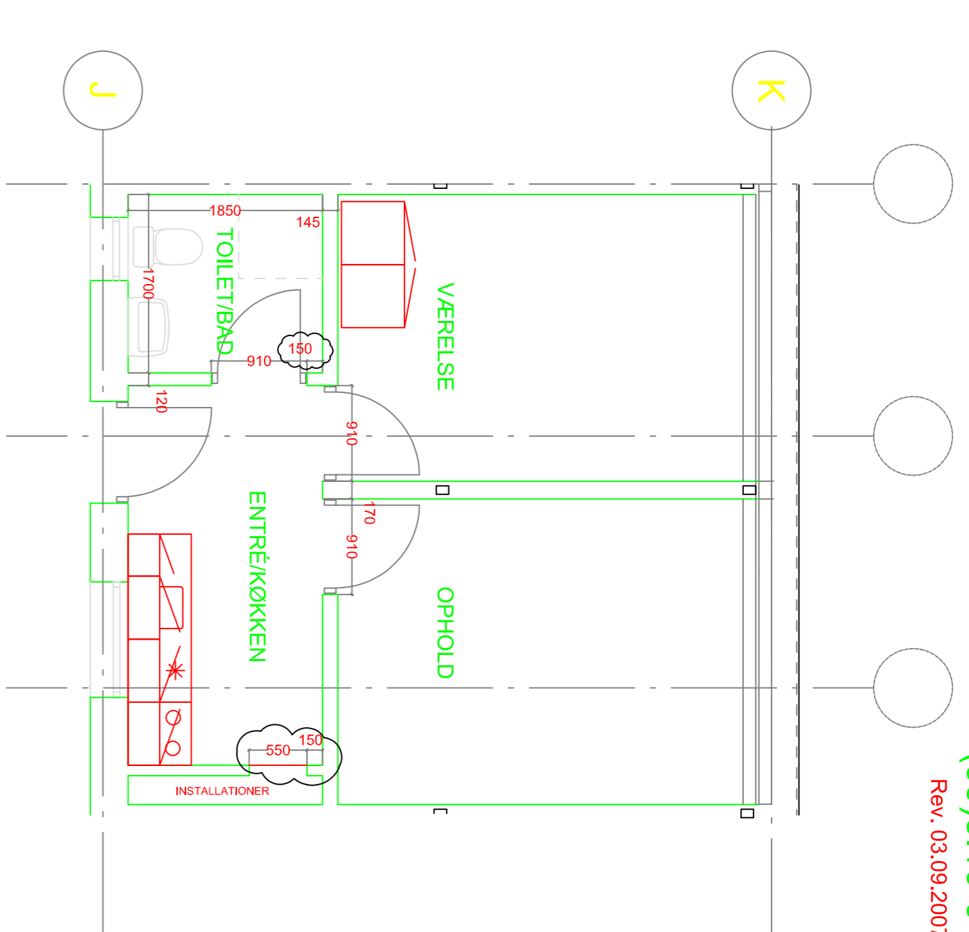
LEJLIGHEDSTYPE D 1½ VÆRELSE
