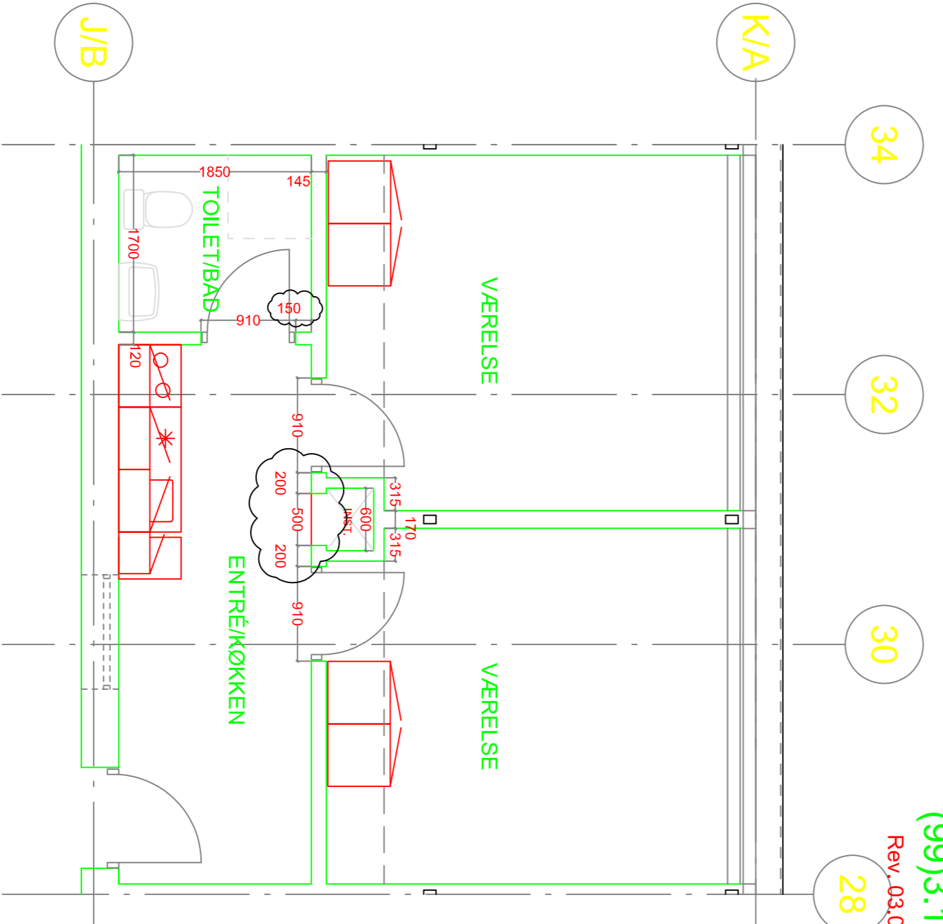
LEJLIGHEDSTYPE F DUBLETTER
