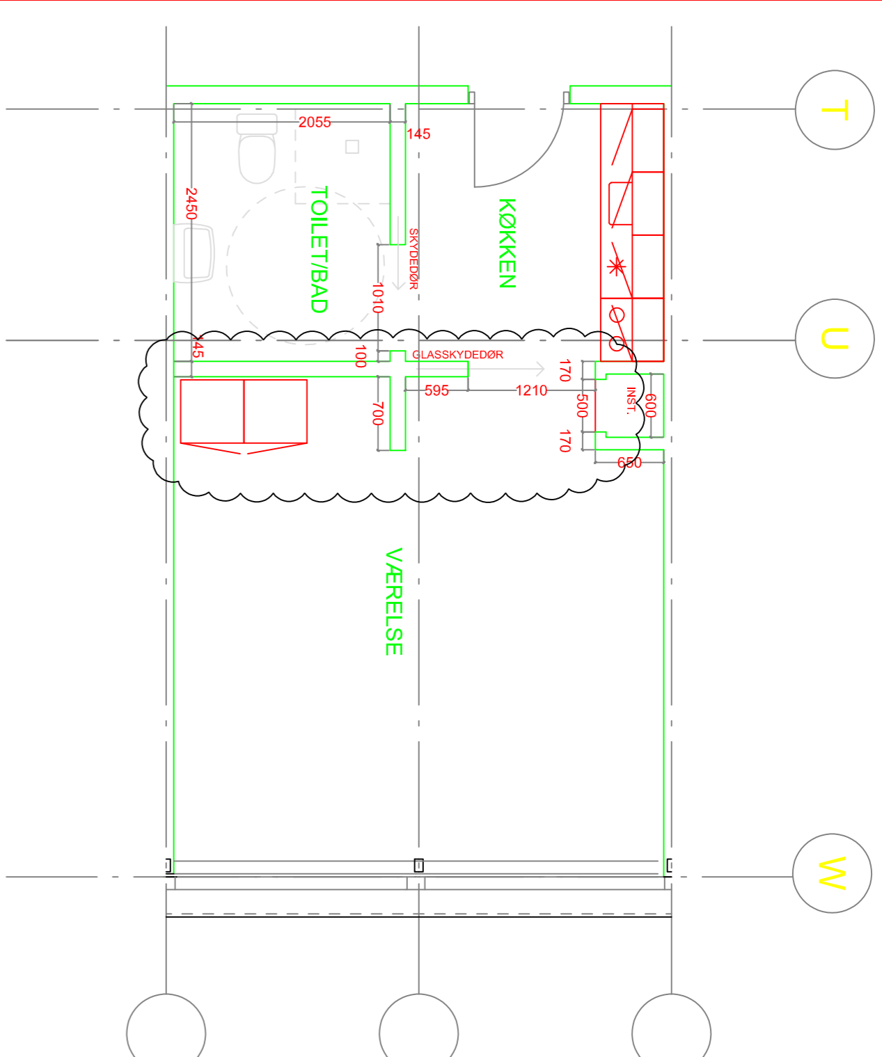
LEJLIGHEDSTYPE C 1 VÆRELSE (HANDICAPENET)
