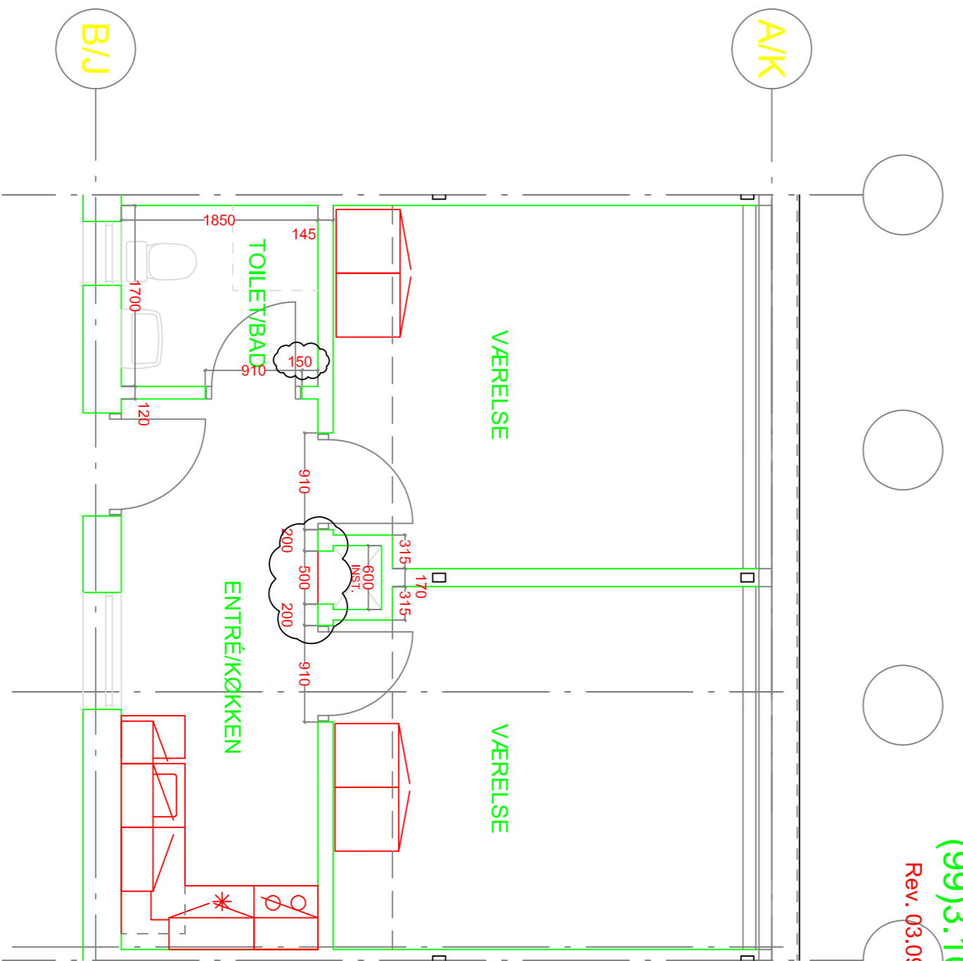
LEJLIGHEDSTYPE E DUBLETTER
