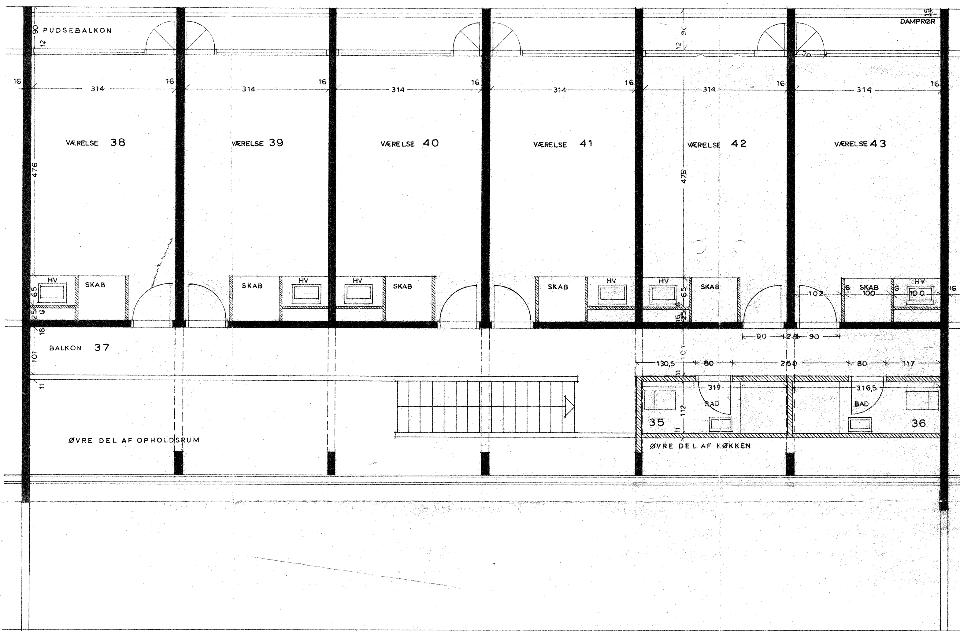
2. ETAGE
