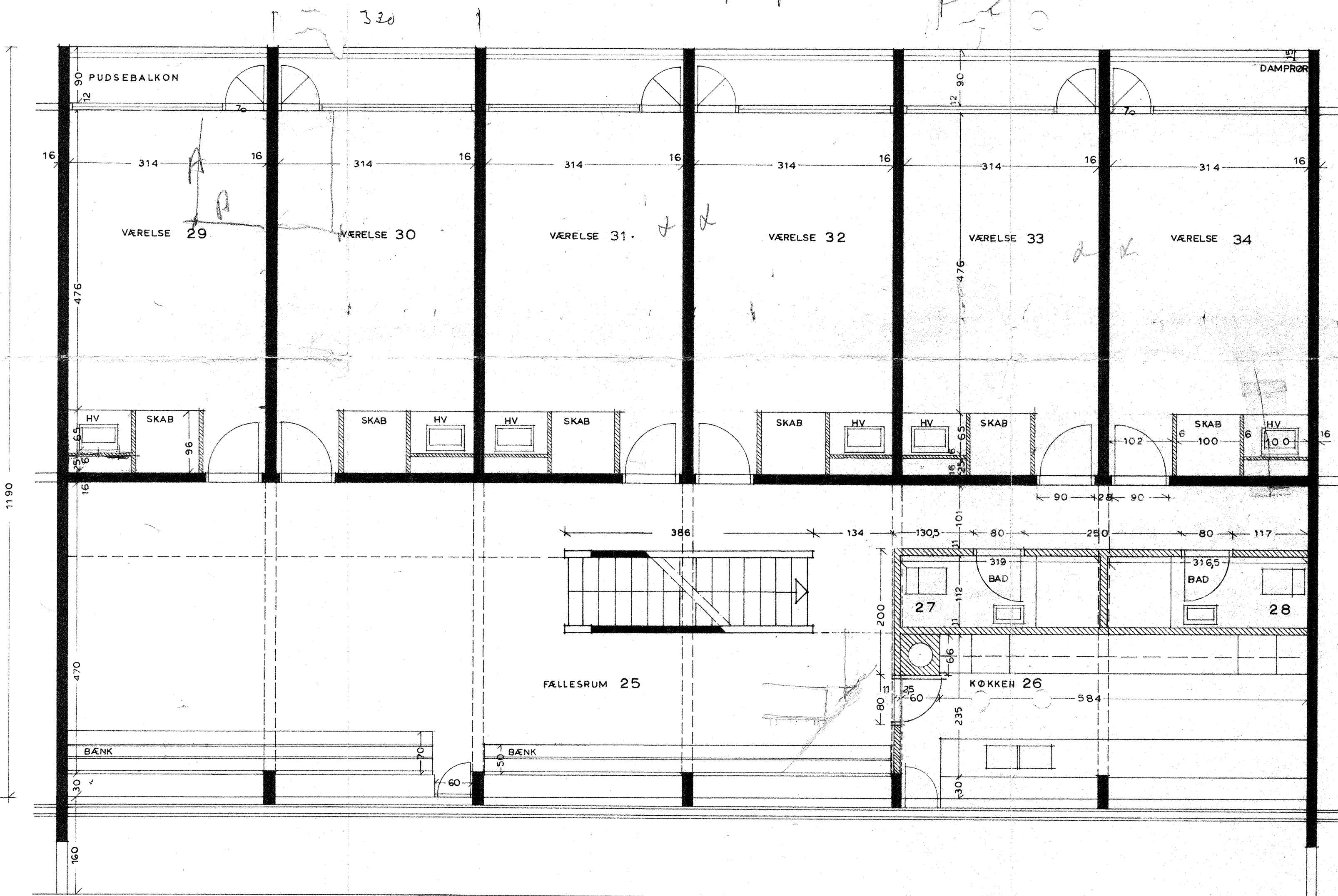
1. ETAGE
